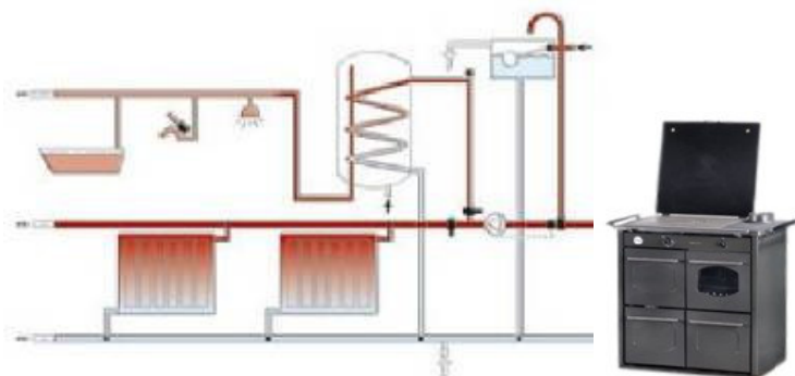
Schéma de principe d'une installation de chauffage et eau chaude, alimentée par un appareil fonctionnant au bois
